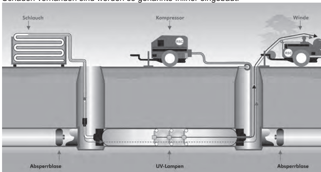
Abbildung 4: Schema zur Inlinersanierung (UV-Liner)
