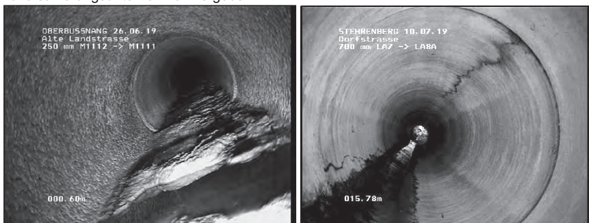
Abbildung 2: Beispiele von Schäden; Harte Ablagerungen (links) und Riss im Rohrscheitel (rechts)
